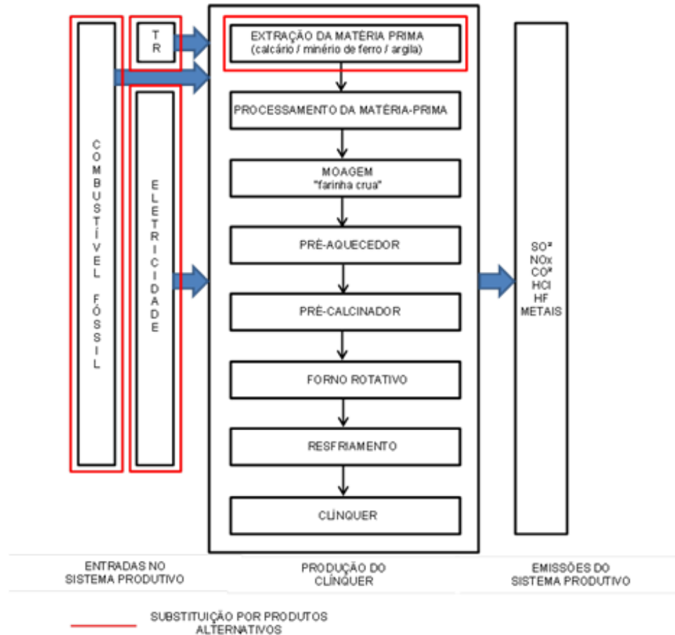
Figura 02: Limites do sistema para a análise do berço ao portão da fábrica da produção do clínquer com o apontamento das possíveis inserções de alternativas no processo produtivo.
