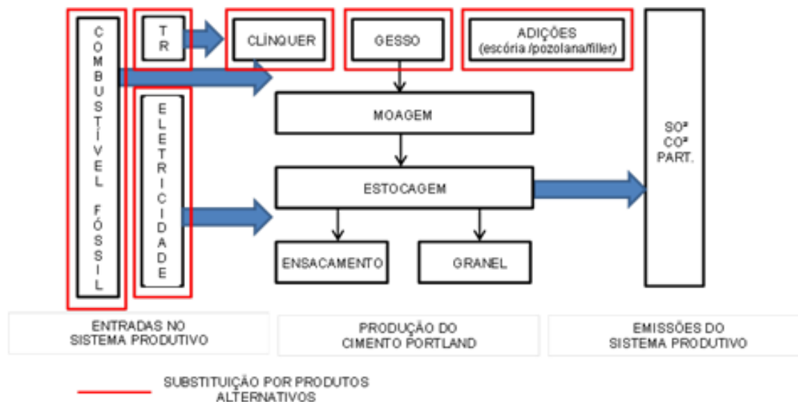
Figura 03: Limites do sistema para a análise do berço ao portão da fábrica da produção do Cimento Portland com o apontamento das possíveis inserções de alternativas do processo produtivo
