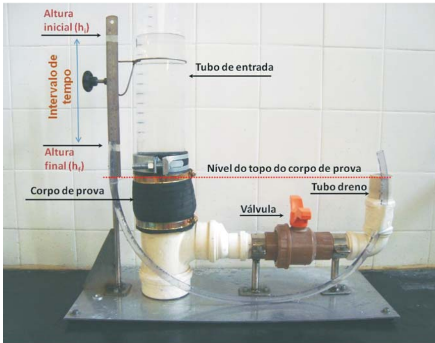
Figura 10 - Permeômetro de carga variável para determinação do coeficiente de permeabilidade do concreto poroso
